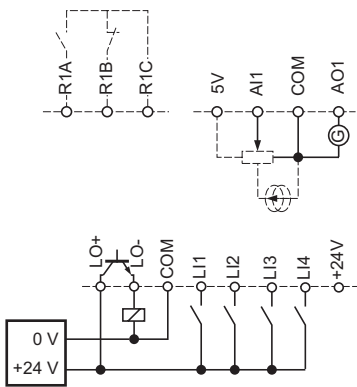
源型 - 使用外部电源
