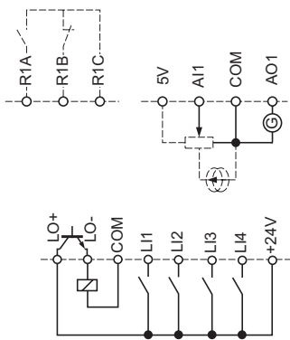
源型 - 使用内部电源
