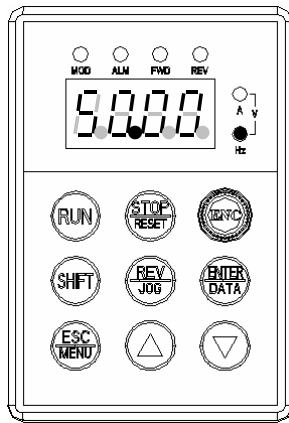
图 c 运行状态，显示运行状态参数
