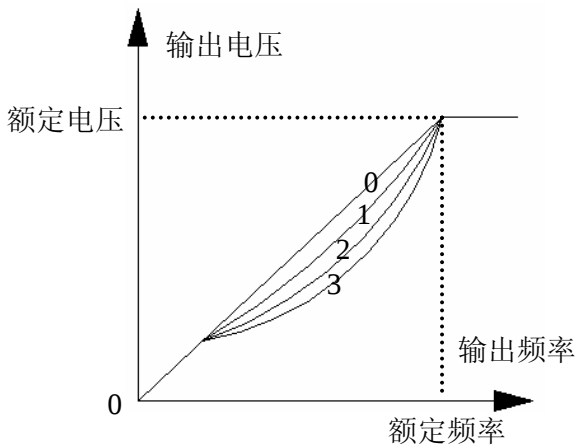
图 6-5 V/F 曲线
