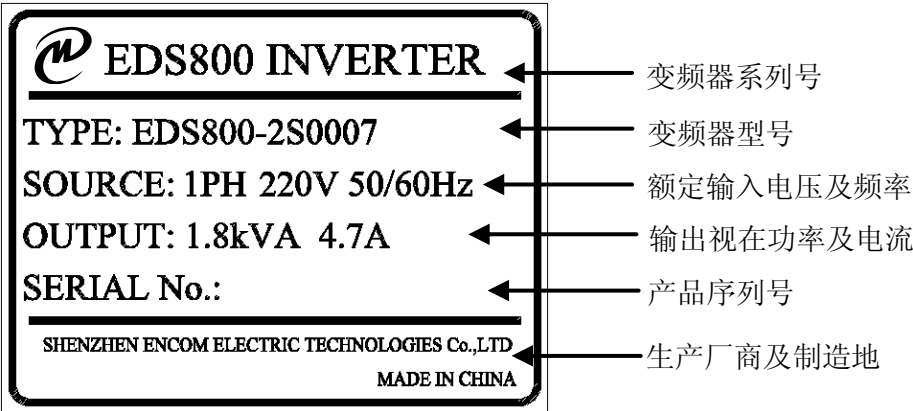
图 2-2 变频器铭牌
