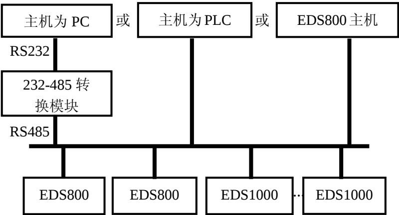
图 10-1 组网方式示意图
