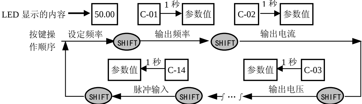
图 4-6 待机状态参数显示操作示例
