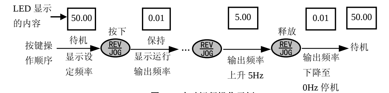
图 4-9 点动运行操作示例
