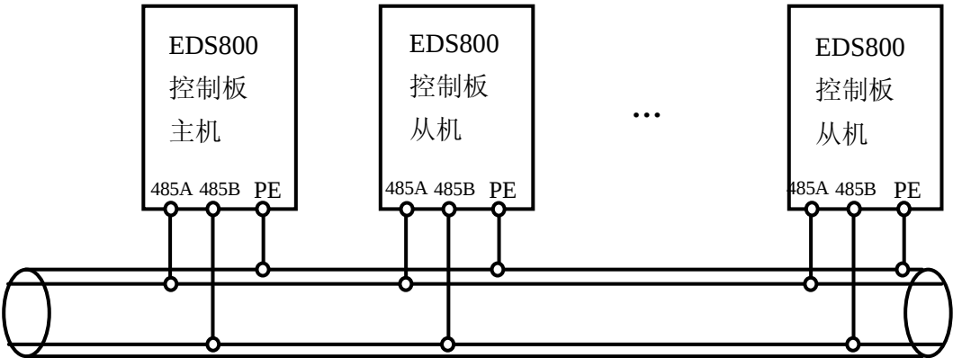
图 3-13 变频器多机通信时推荐的接线图(变频器、电机全部良好接地)
