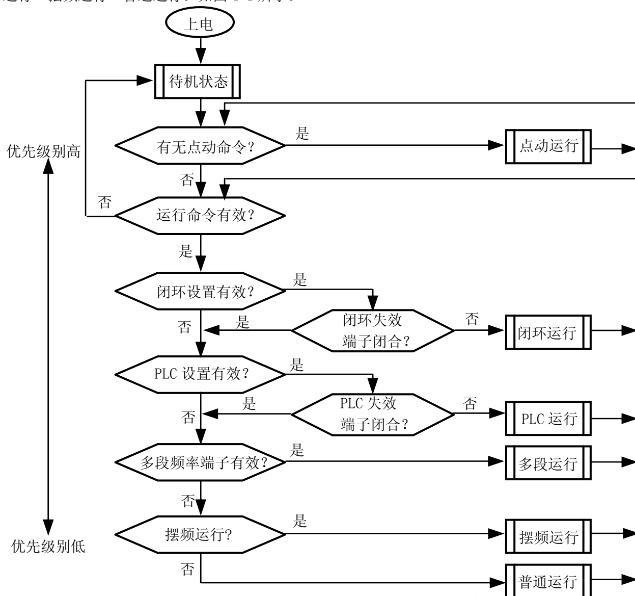
图 4-1 EDS800 变频器运行状态的逻辑程序
