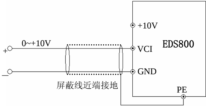
图 3-8 VCI 端子配线图
