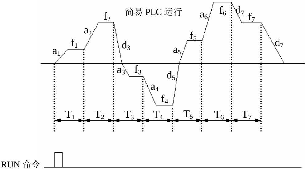
图 6-21 PLC 单循环后停机方式
