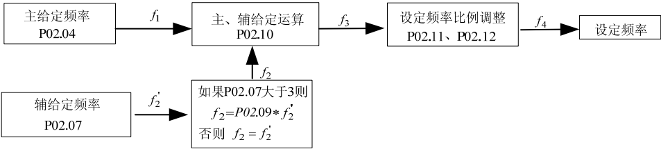
图6-5 设定频率合成示意图
