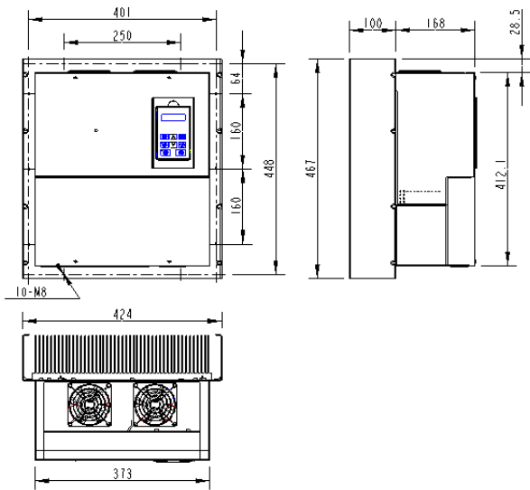
图1-5 穿墙安装之 WR6 外形及安装尺寸示意图
