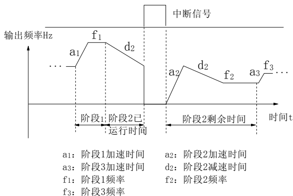
图6-65 PLC 起动方式 2
