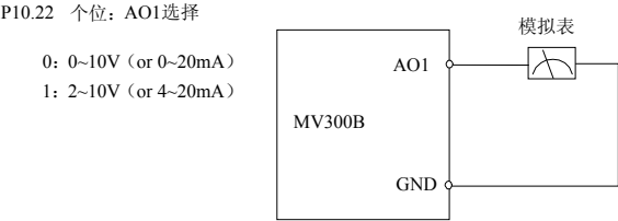
图3-8 模拟输出端子配线
