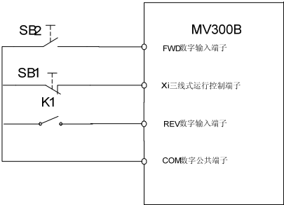
图6-29三线式运转模式 2
