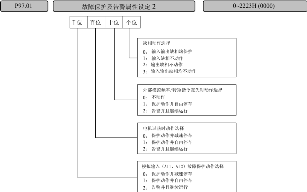
图6-75 故障保护及告警属性设定 2
