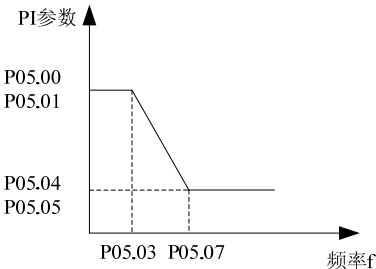
图6-14 PI 参数示意图
