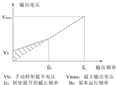
图6-22 转矩提升（提升量为阴影部分）
