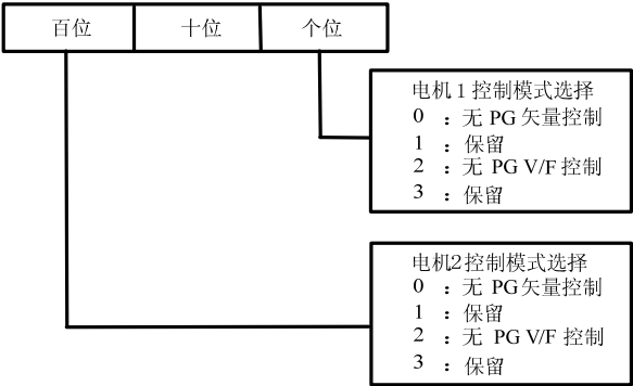
图6-6 电机控制模式图
