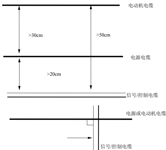
图3-25 系统配线要求
