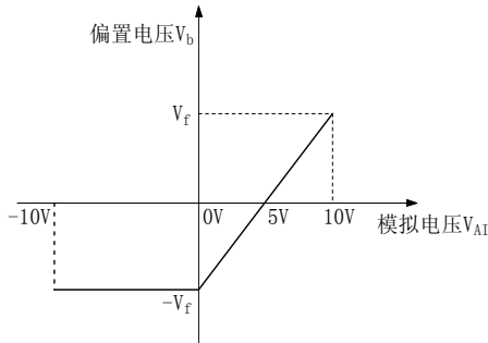
图6-44 输出电压偏置
