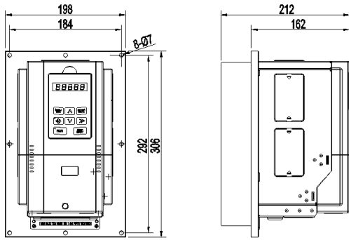
图1-2 WR3 外形及安装尺寸示意图
