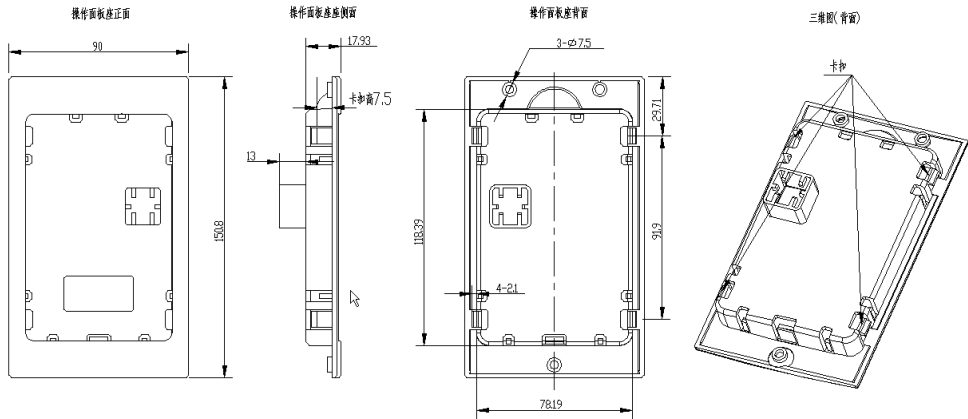
图1-11 操作面板固定座外形尺寸
