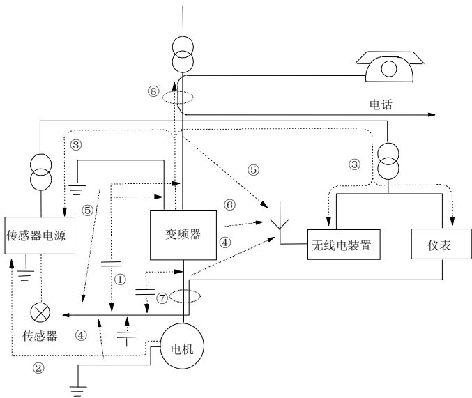
图3-24 噪声传播路径示意图
