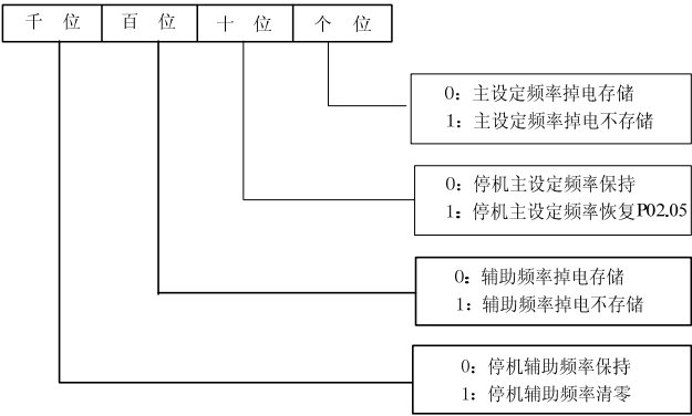
图6-8 数字频率控制 LED 设定
