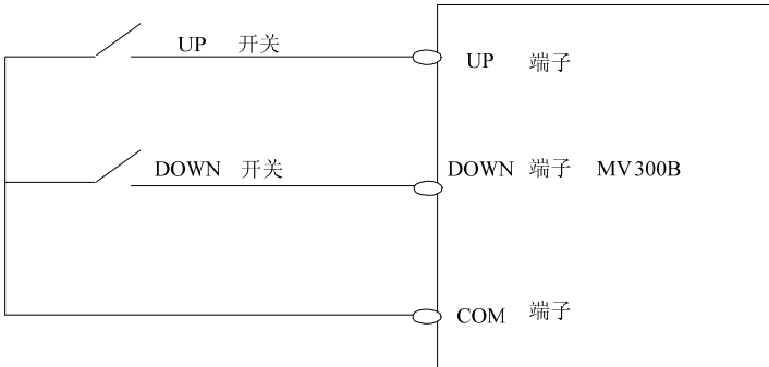
图6-7 数字设定 2 方式时接线示意图
