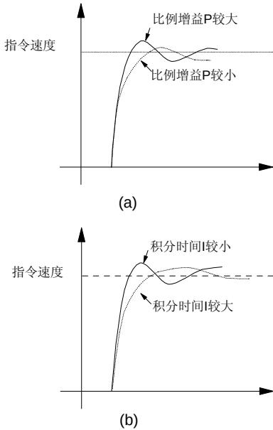
图6-16 阶跃响应与 PI 关系图
