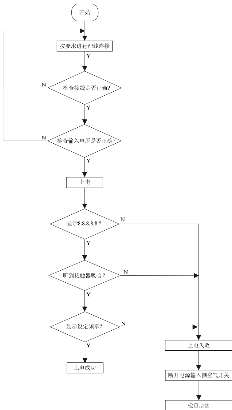
图4-10 变频器首次上电操作流程
