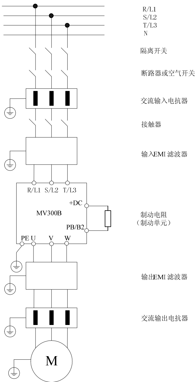
图3-2 变频器与选配件的连接
