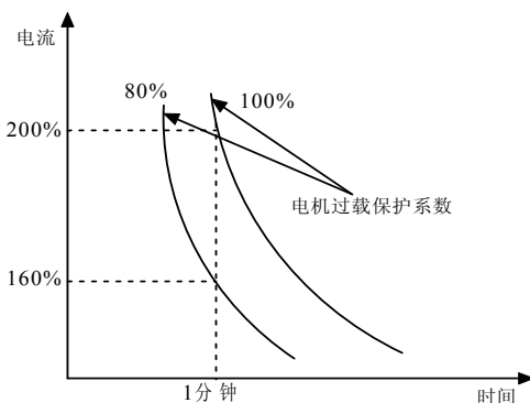
图6-13 电机过载保护系数设定
