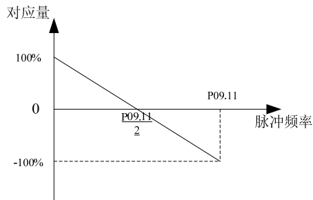
图6-31 中心点模式 1
