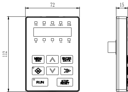
图1-10 操作面板的外形和安装尺寸
