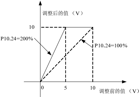
图6-49 模拟输出与增益关系曲线
