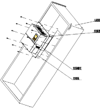
带安装板的变频器正面安装
