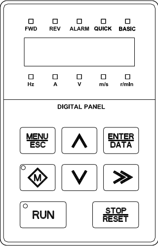
图4-1操作面板示意图
