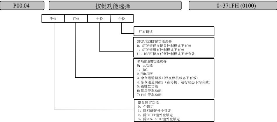
图6-1 按键功能选择
