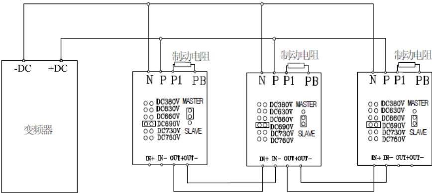
图附 2-2 变频器与制动组件连接图
