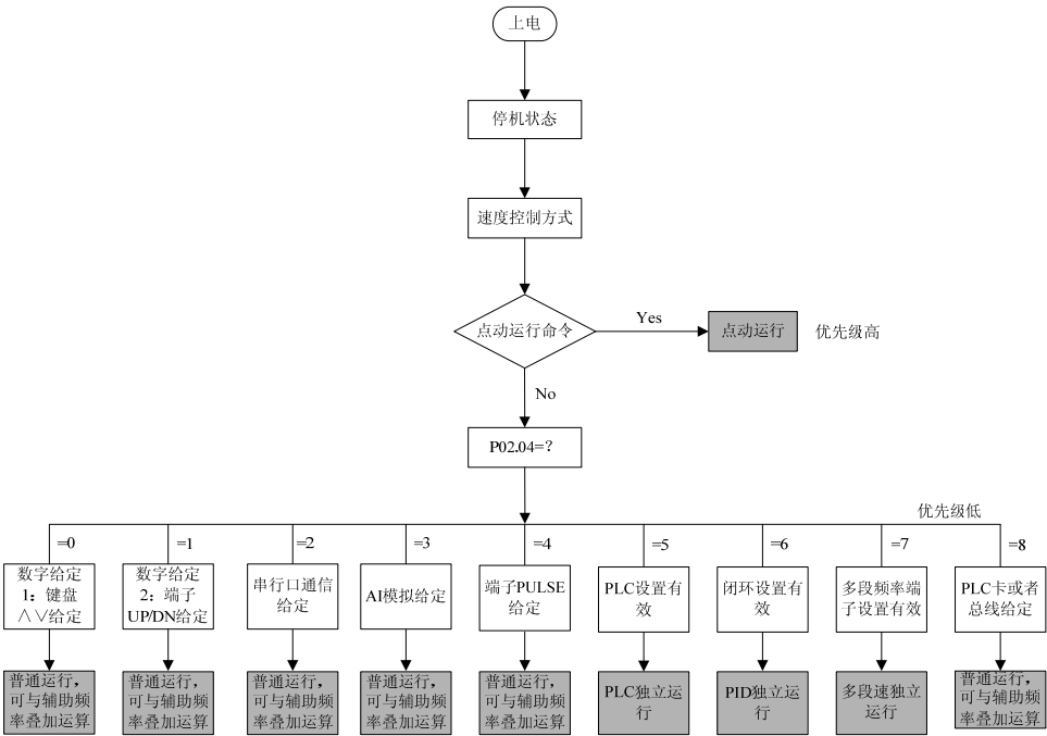
图4-9 速度控制模式下运行方式选择
