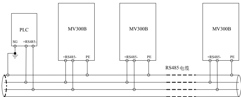
图3-11 PLC与变频器多机通讯时推荐的接线图（变频器、电机全部良好接地）
