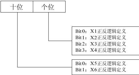
图6-33 端子正反逻辑设定
