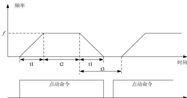
图6-56 点动运行参数说明
