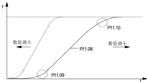
图6-54 S 曲线调整示意图说明
