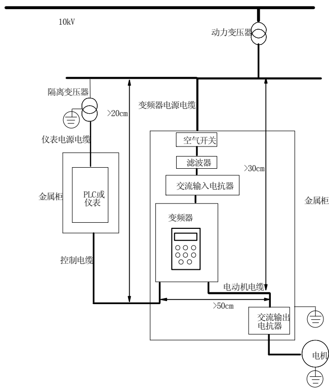
图3-35 变频器的安装示意图
