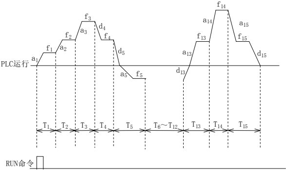
图6-61 PLC 单循环后停机方式
