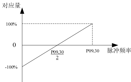
图6-39 中心点模式 2
