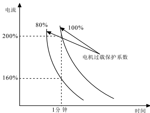
图6-11 电机过载保护系数设定
