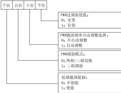
图6-58 PWM 模式优化选择
