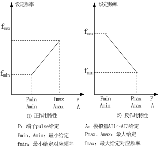
图6-41 模拟输出频率特性曲线
