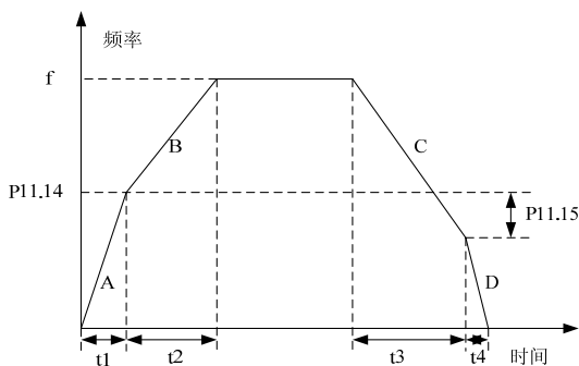
图6-55 加减速时间 1、2 切换示意图
