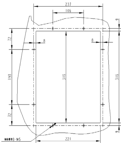
图1-7 穿墙安装之 WR4 的机柜开孔和铆螺母尺寸示意图
