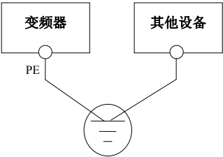
图3-29 接地示意图 2
