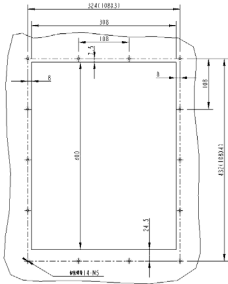
图1-8 穿墙安装之 WR5 开孔及铆螺母尺寸示意图
