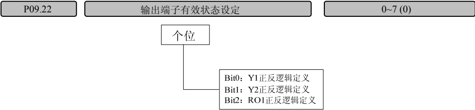
图6-34 输出端子有效状态设定
