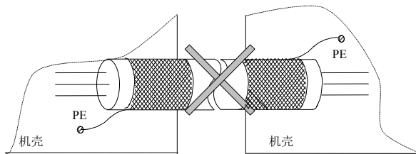
图3-27 错误的屏蔽接地方法
