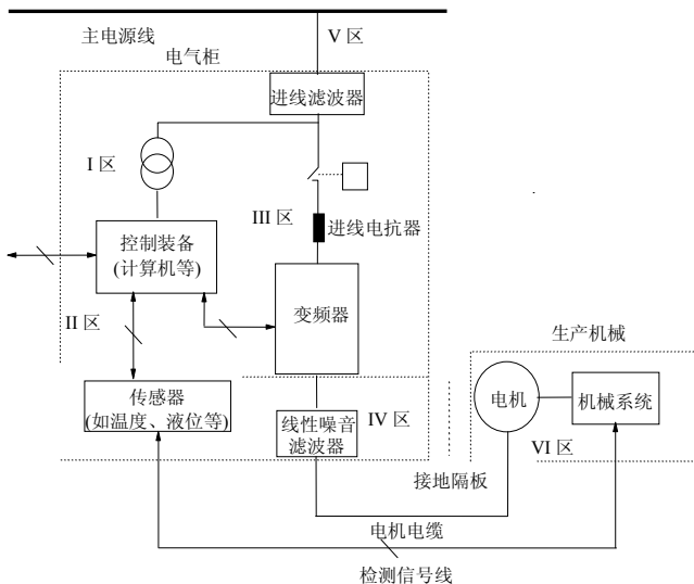
图3-34 变频器 EMC 安装推荐区域划分示意图
