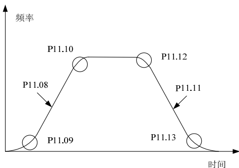
图6-53 S 曲线参数示意图
