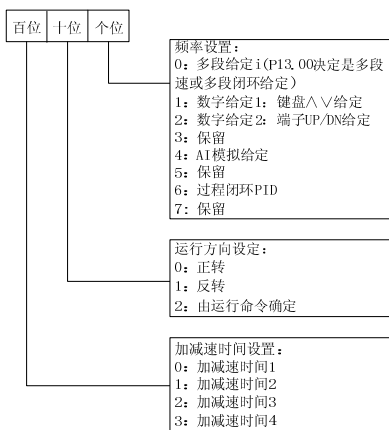
图6-66 PLC 起动方式 2
