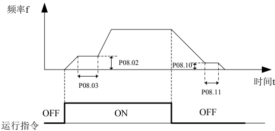
图6-23 启动时/停止时 DWELL 功能时序图
