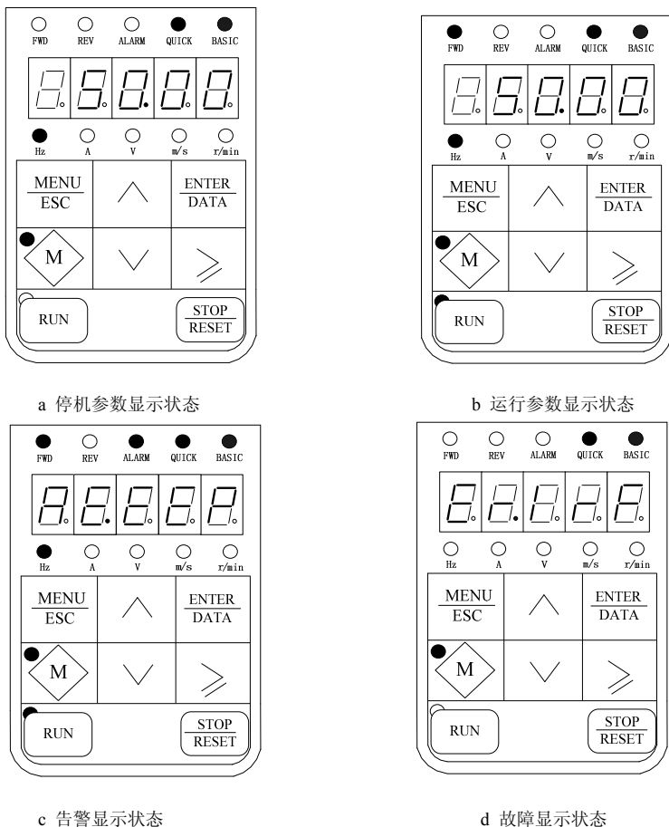
图4-2 变频器停机、运行、告警、故障时的显示
