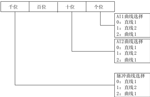
图6-46 模拟、脉冲曲线选择
