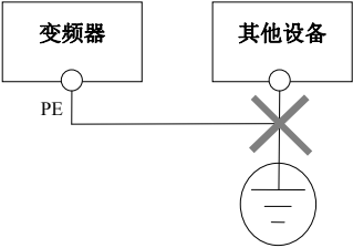
图3-30 接地示意图 3
