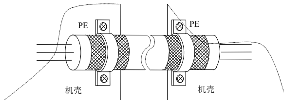
图3-26 正确的屏蔽接地方法
