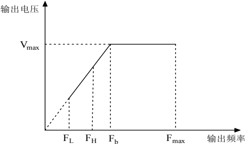
图6-9 极限频率参数定义示意图
