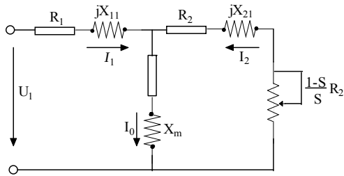
图6-10 异步电机稳态等效电路图
