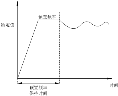
图6-69 PID 预置频率运行示意图
