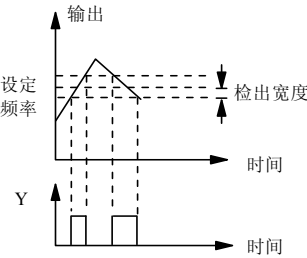
图6-35 频率到达信号输出示意图
