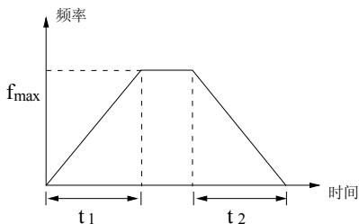
图6-51 直线加减速
