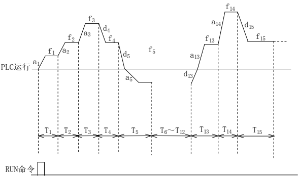
图6-62 PLC 单循环后保持方式
