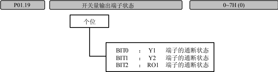
图6-4 开关量关输出端子状态
