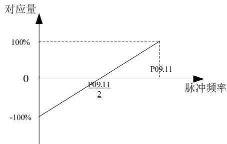
图6-32 中心点模式 2
