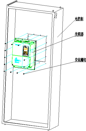
图2-2 变频器的正面安装方式（以 VR5 为例）
