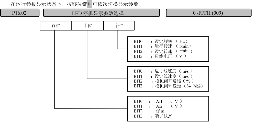
图6-73 LED 停机显示参数选择设定
