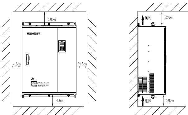
图2-5 55kW H/75kW N 及以上产品安装间隔距离
