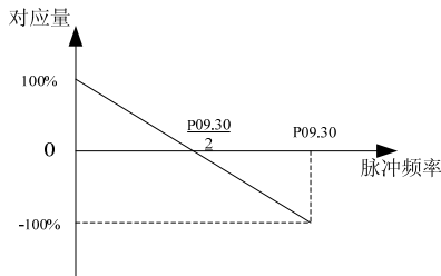
图6-38 中心点模式 1
