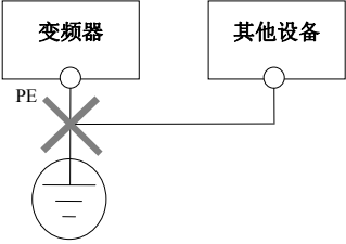
图3-31 接地示意图 4
