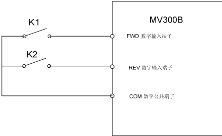
图6-26 两线式运转模式 1
