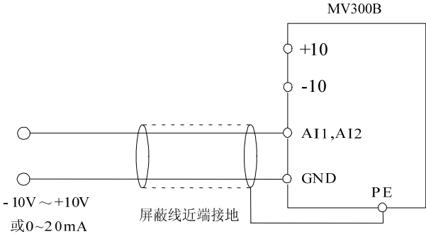
图3-7 AI1、AI2 端子端子配线图
