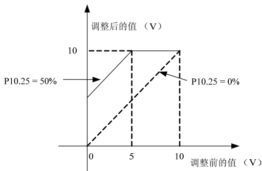
图6-50 模拟输出与零偏关系曲线
