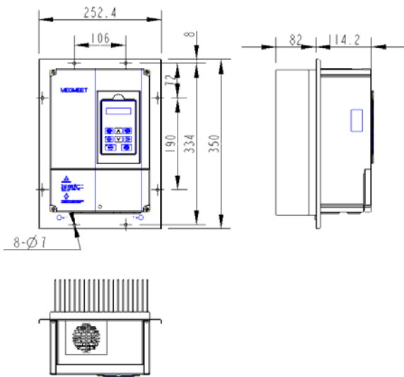
图1-3 穿墙安装之 WR4 外形及安装尺寸示意图
