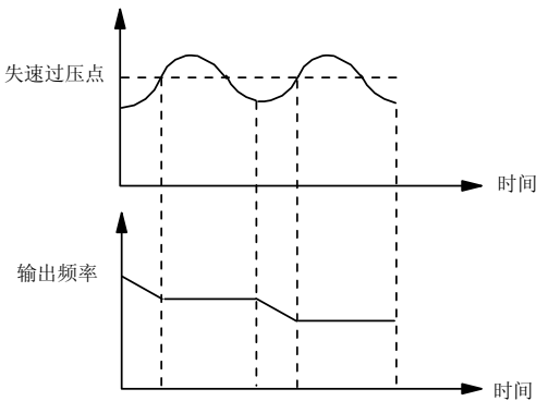
图6-79 过压失速功能
