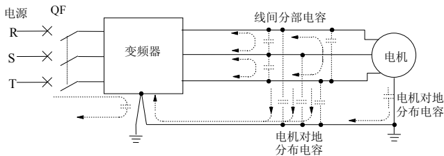
图3-33 漏电流路径
