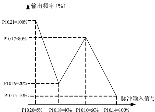
图6-47 脉冲信号输入实例参数设置
