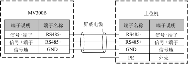
图3-9 RS485-RS485 通讯配线
