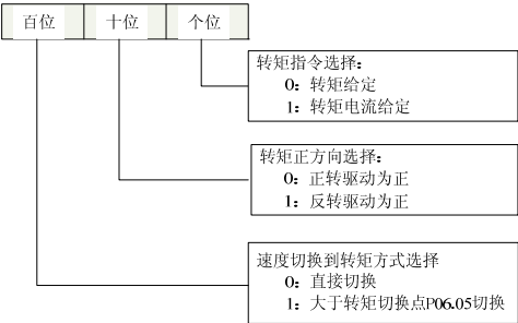
图6-19 转矩控制模式
