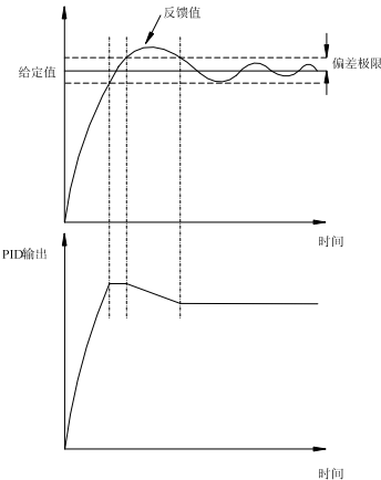
图6-68 偏差极限示意图
