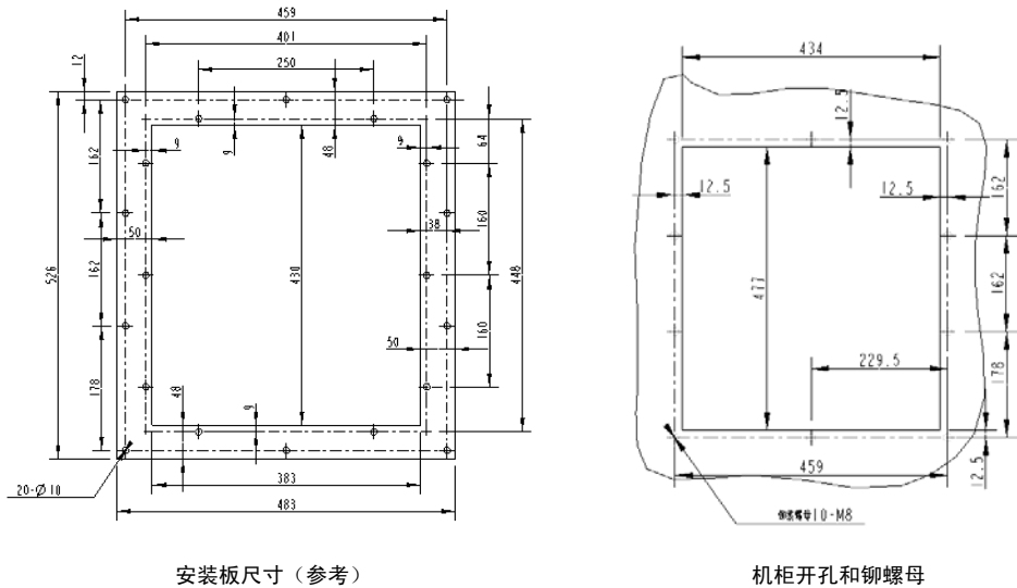
图1-9 从机柜正面安装之 WR6 安装板尺寸和机柜开孔尺寸示意图
