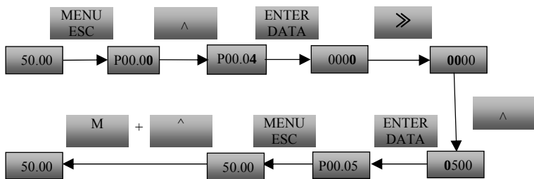
图4-4 操作面板按键锁定的操作示例
