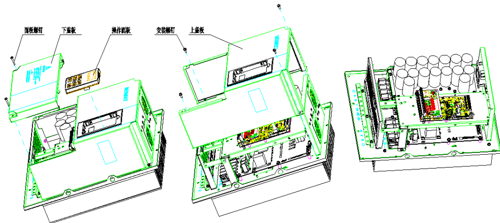
图2-1 变频器部件的拆卸安装示意图（以 WR5 为例）
