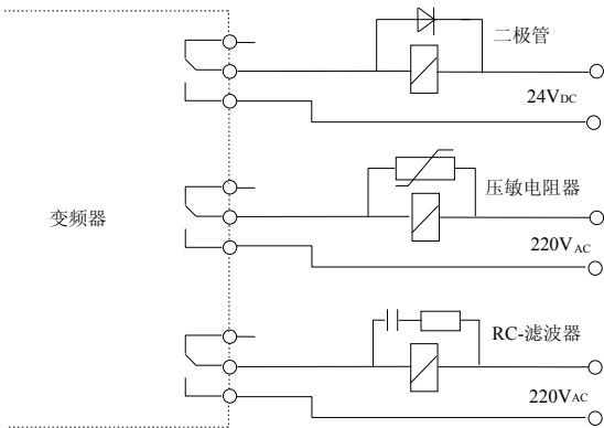
图3-32 继电器、接触器及电磁制动器要求
