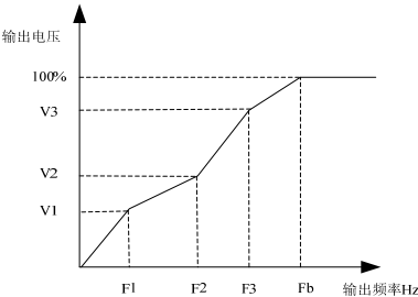
图6-21 多段 V/F 曲线
