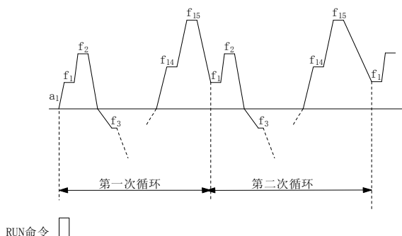
图6-63 PLC 连续循环方式
