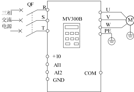
图3-1 主回路简单配线图
