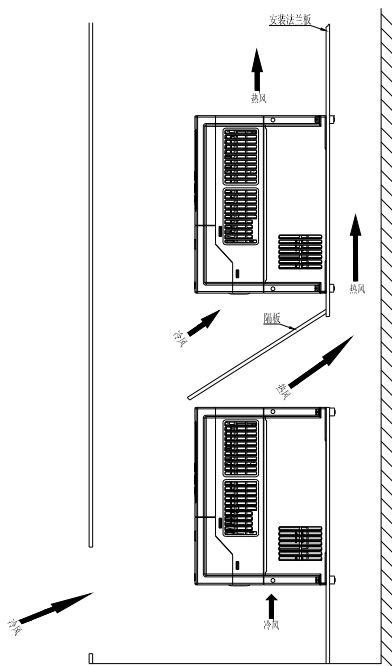
图2-6 两台变频器以上的安装
