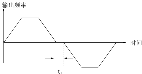
图6-25 正反转死区时间
