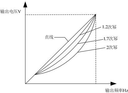
图6-20 V/F 曲线
