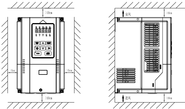
图2-4 45kW H/55kW N 及以下产品安装间隔距离
