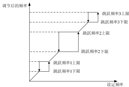
图6-57 跳跃频率及范围示意图
