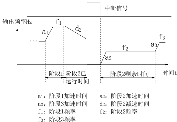
图6-64 PLC 起动方式 1
