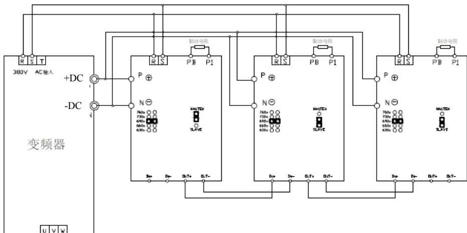
图附 2-3 变频器与制动组件连接图
