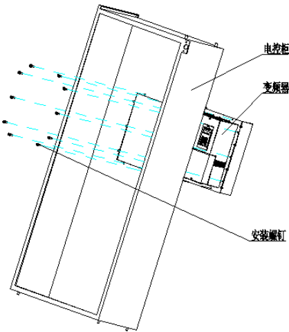
变频器的背面安装
