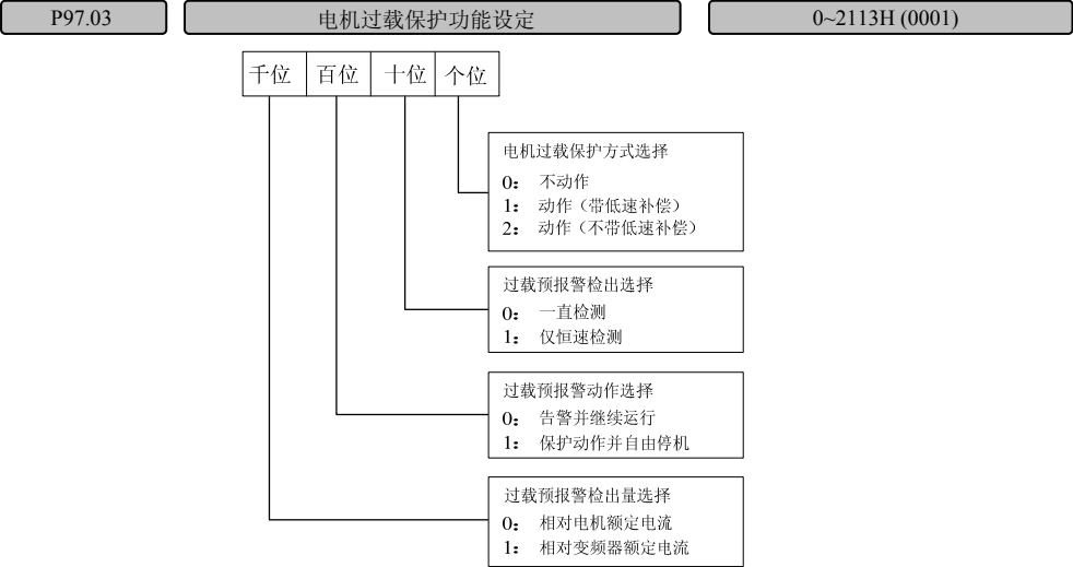
图6-77 电机过载保护功能设定
