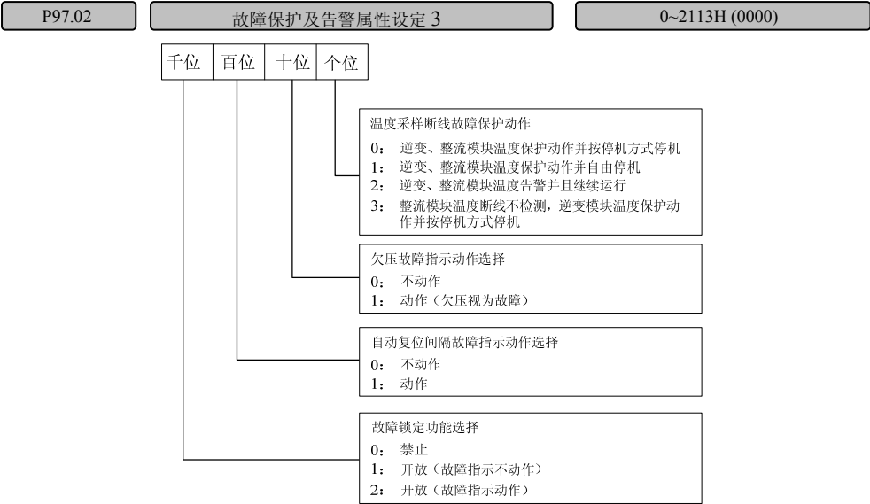
图6-76 故障保护及告警属性设定 3
