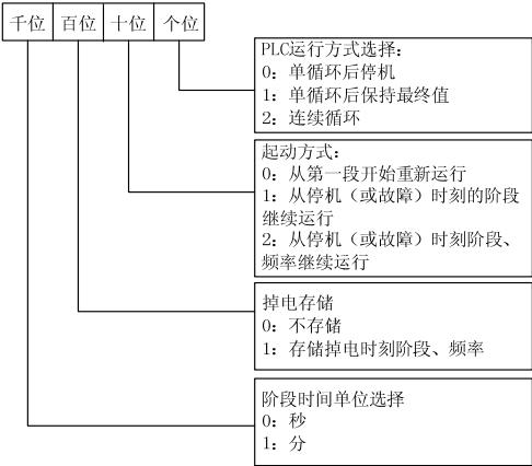
图6-60 简易 PLC 运行方式选择
