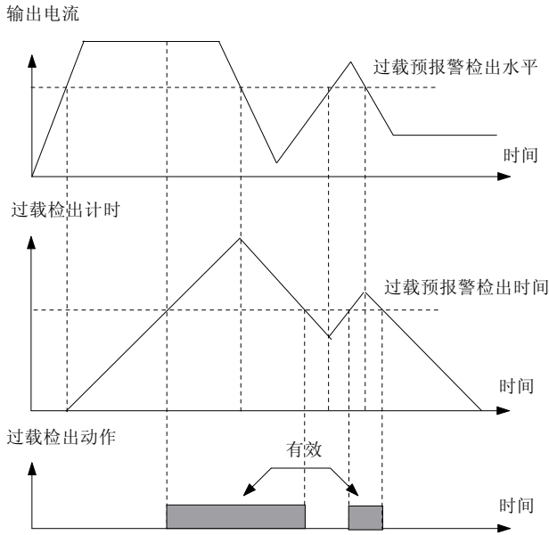
图6-78 过载预告警检出功能示意图
