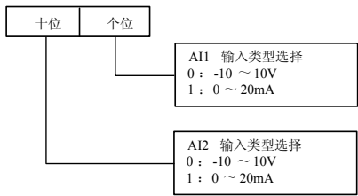
图6-42 模拟输入类型选择
