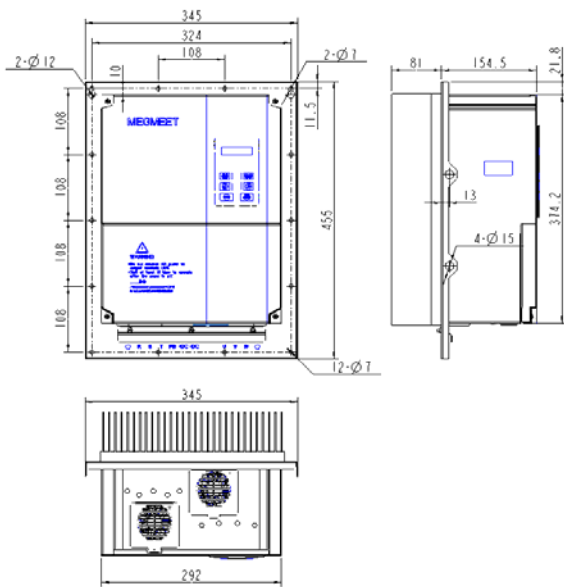
图1-4 穿墙安装之 WR5 外形及安装尺寸示意图
