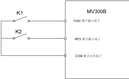
图6-27 两线式运转模式 2
