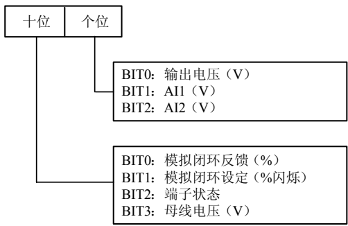
图6-72 LED 运行显示参数选择 2 设定
