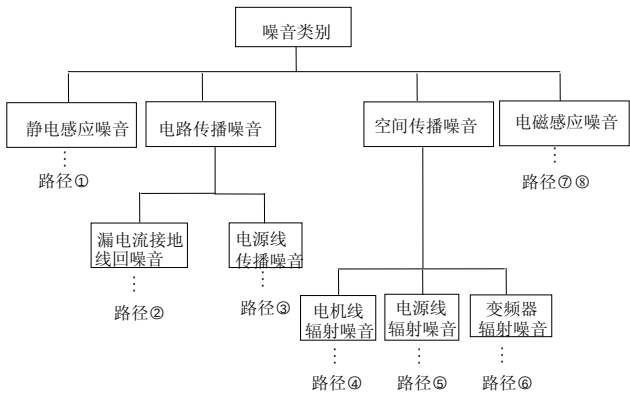
图3-23 噪声分类示意图
