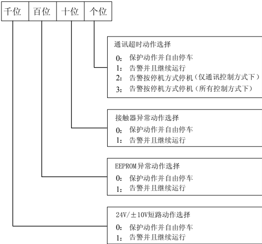
图6-74 故障保护及告警属性设定 1
