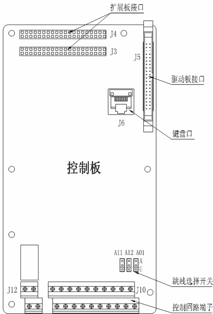
图3-22 控制板示意图
