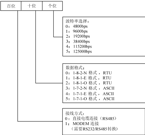
图6-70 通讯配置设定
