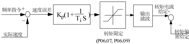
图6-15 速度调节器简化图
