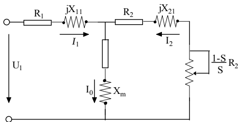
图6-12 异步电机稳态等效电路图
