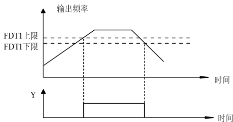
图6-36 频率水平检测示意图
