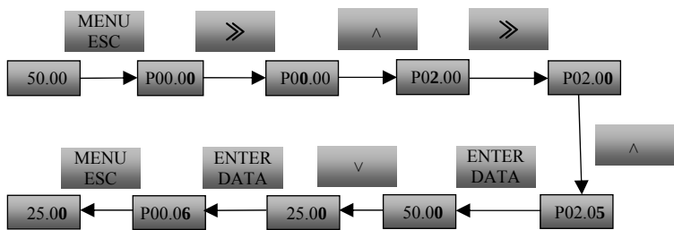
图4-7 设置设定频率操作示例
