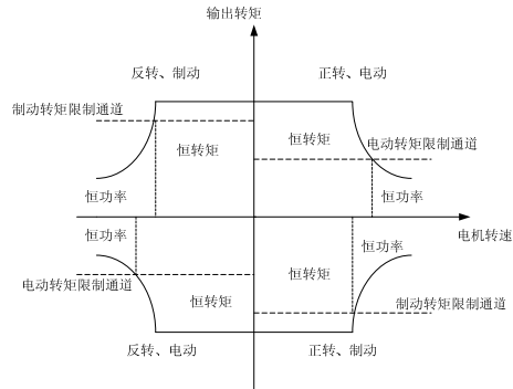
图6-18 转矩控制图
