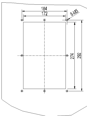
图1-6 穿墙安装之 WR3 的机柜开孔尺寸示意图
