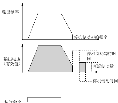
图6-24 减速停车+直流制动示意图
