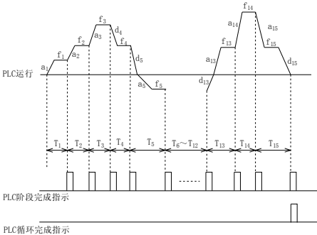
图6-59 简易 PLC 运行图
