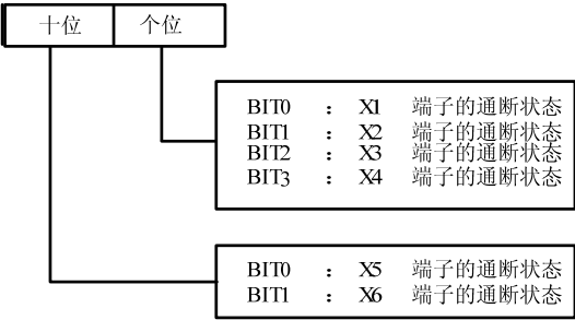
图6-3 开关量输入端子状态
