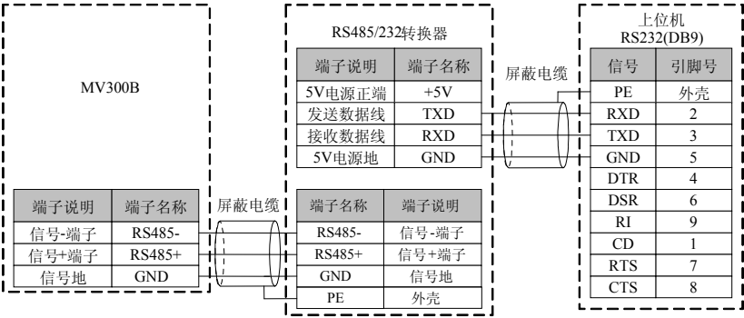
图3-10 RS485-(RS485/232)-RS232 通讯配线
