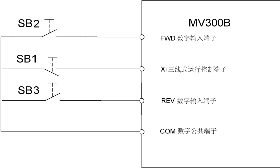
图6-28 三线式运转模式 1
