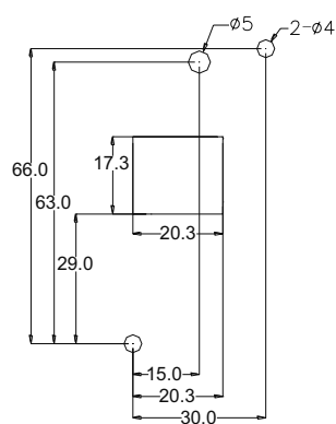
&lt;盘面安装开孔尺寸图&gt;
