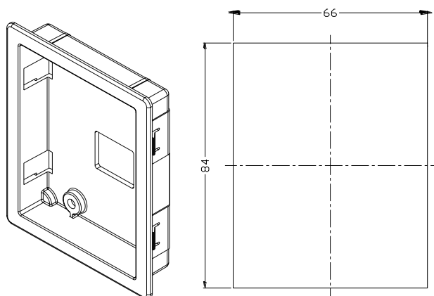
&lt;法兰式安装开孔尺寸图(注)&gt;
