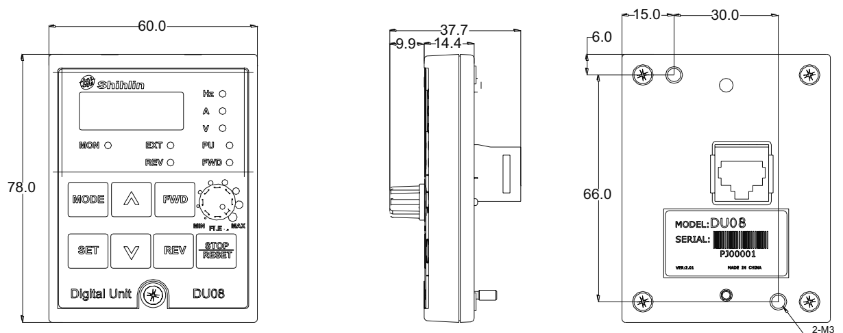
&lt;外形尺寸图&gt;
