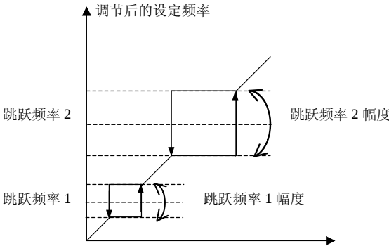
图 6-26 跳跃频率输出
