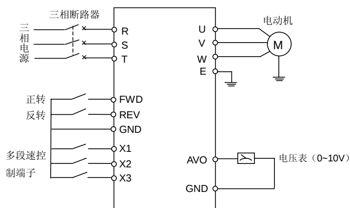
图 9-2 基本接线图
