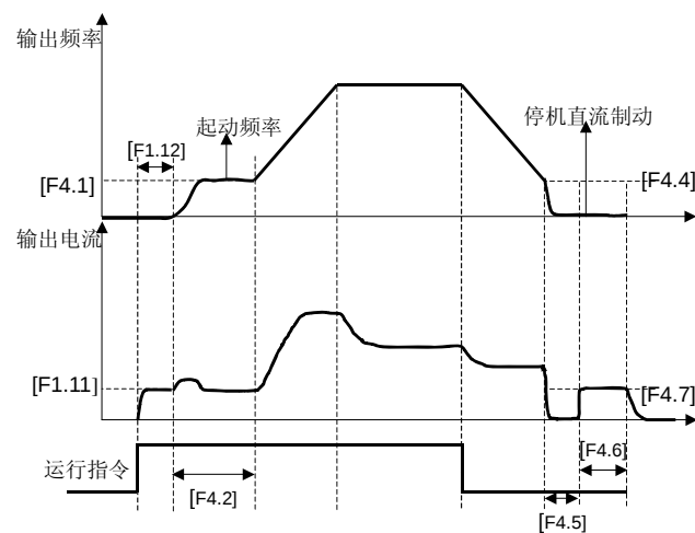
图 6-7 起动与停机过程
