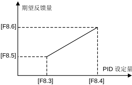
图 6-31 PID 给定量与反馈量的关系
