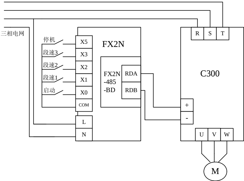
图 2 主回路接线
