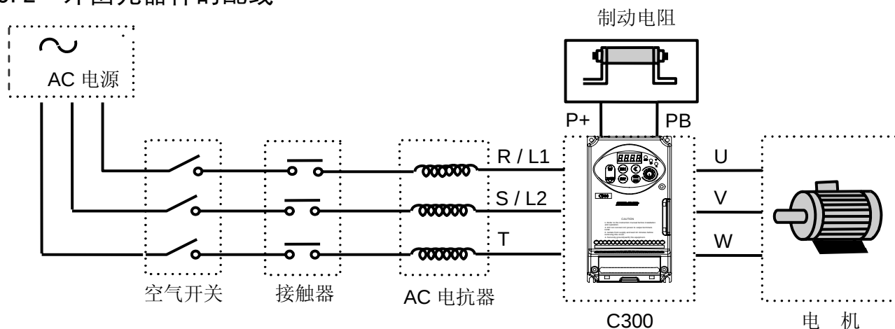
图 3-2 变频器的配线
