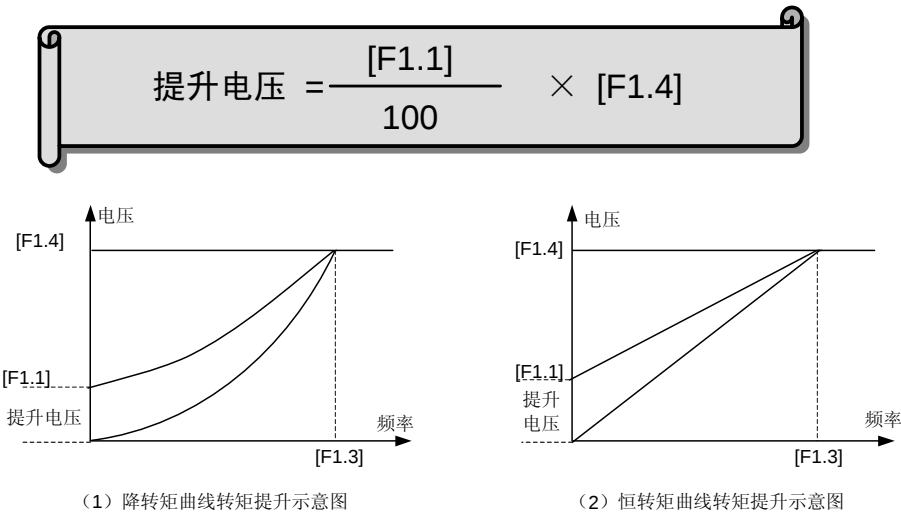
图 6-5 转矩提升
