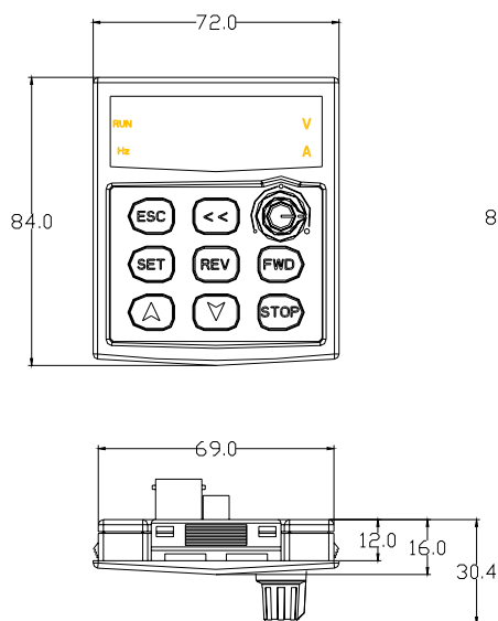
图-D 小操作面板安装底座的尺寸
