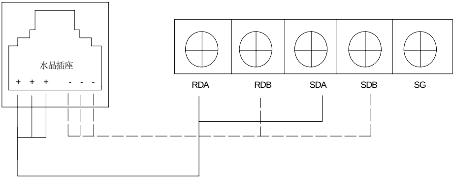
图 1 接线方式
