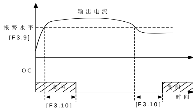
图 6-15 过载报警
