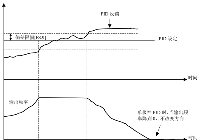
图 6-29 单极性 PID 控制方式
