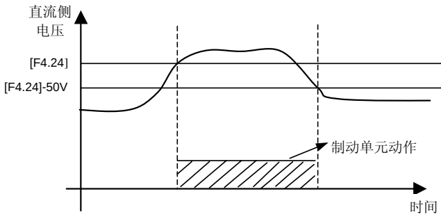
图 6-22 能耗制动
