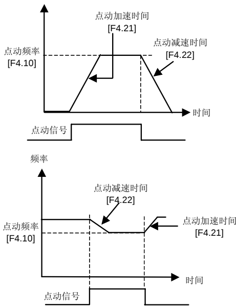
图 6-18 点动运行
