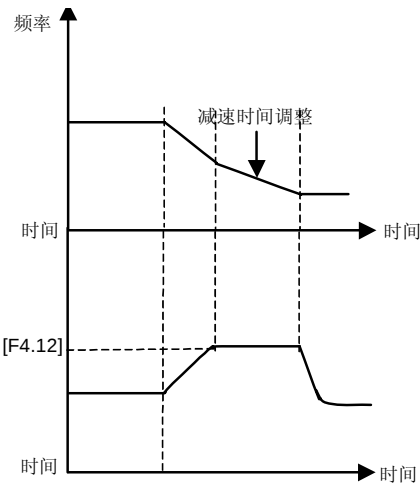
图 6-19 加速力矩与制动力矩示意图
