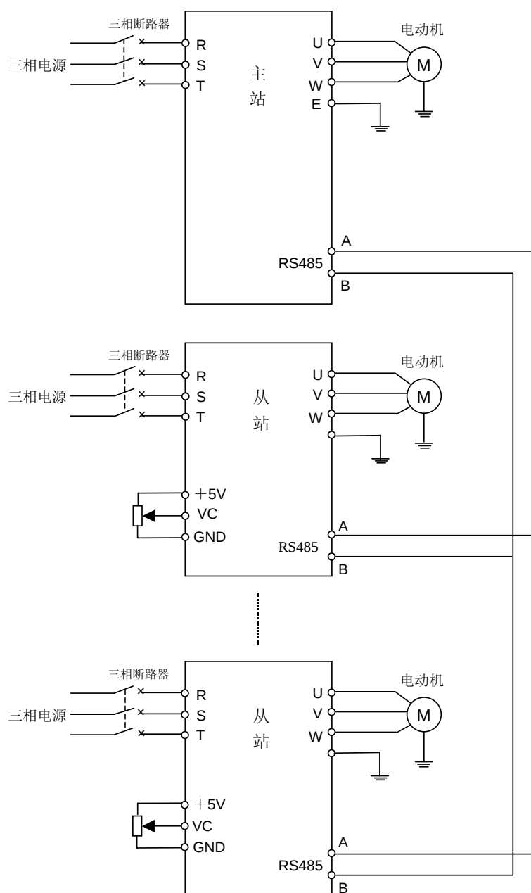
图 9-4 基本接线图
