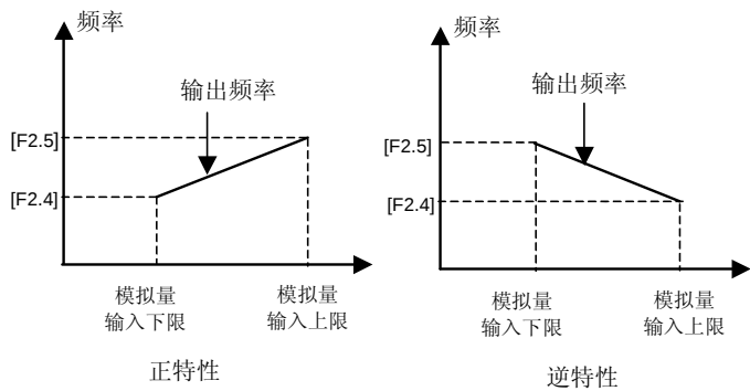
图 6-10 模拟输入与设定频率对应图示
