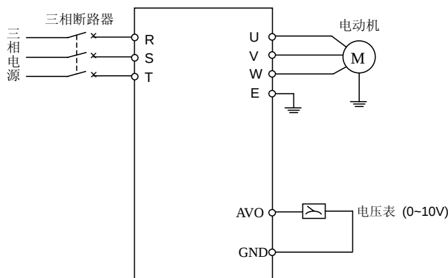
图 9-1 基本接线图
