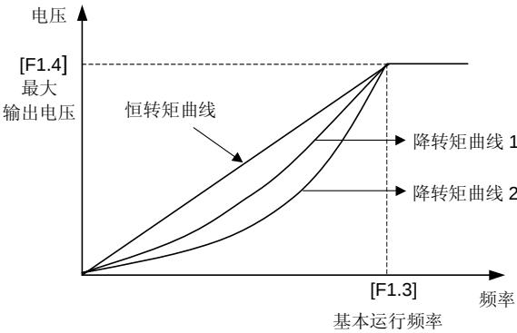
图 6-4 V/F 曲线
