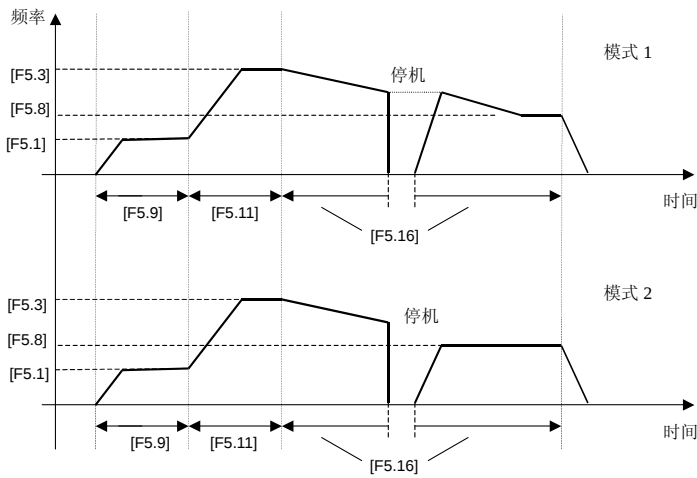
图 6-24 PLC 断点恢复
