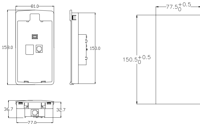
图-A 操作面板安装底座的尺寸
