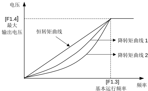
图 6-4 V/F 曲线
