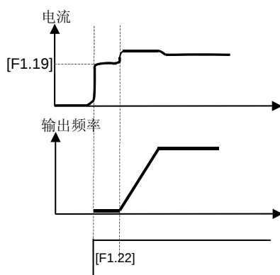
图 6-9 启动预励磁输出
