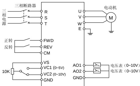
图 9-2 基本接线图
