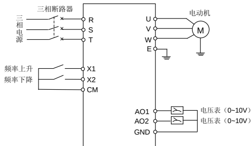
图 9-4 基本接线图
