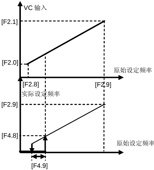
图 6-18 频率输出过零点曲线
