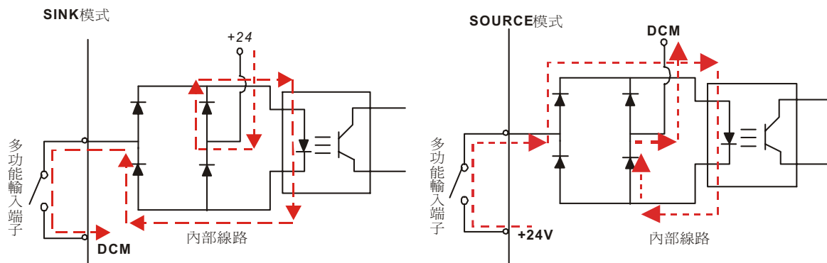
控制端子標示說明
