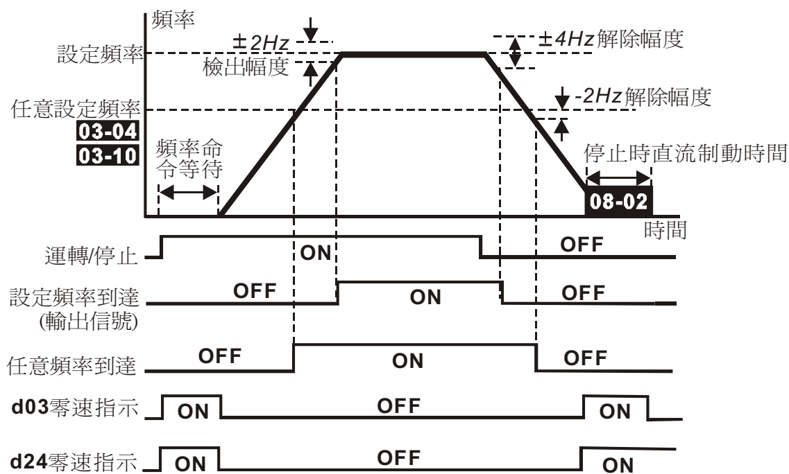
多機能端子與頻率到達輸出時序圖
