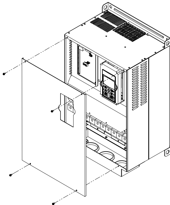
40-100HP/30-75kW(Frame E, E1)
