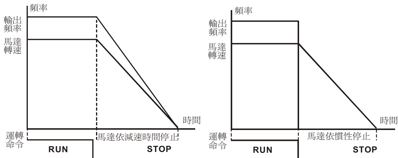
減速停止與自由運轉停止
