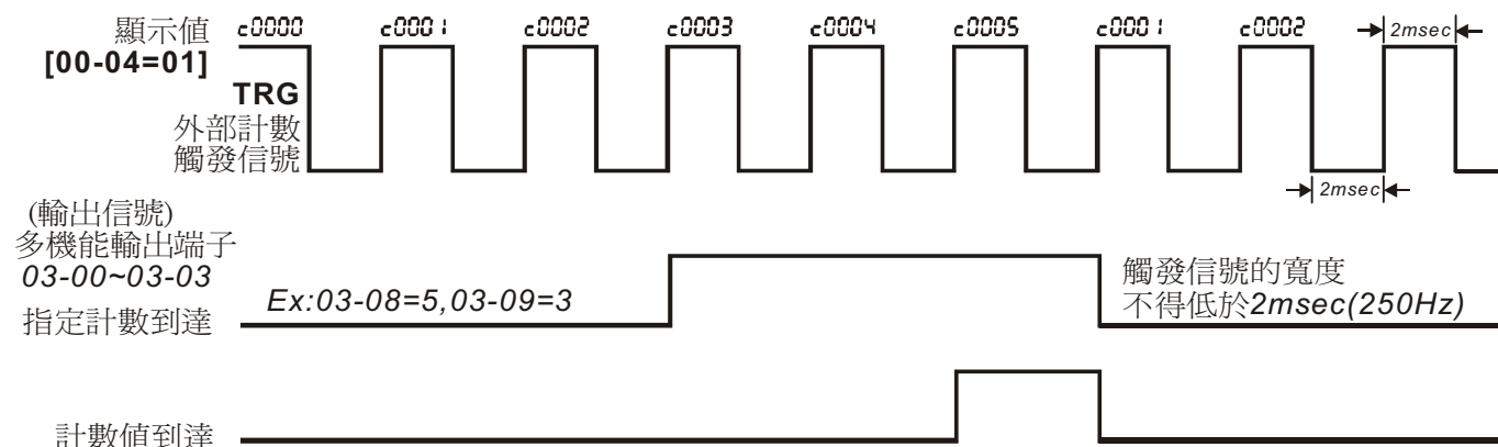
外部計數端子與計數到達時序圖
