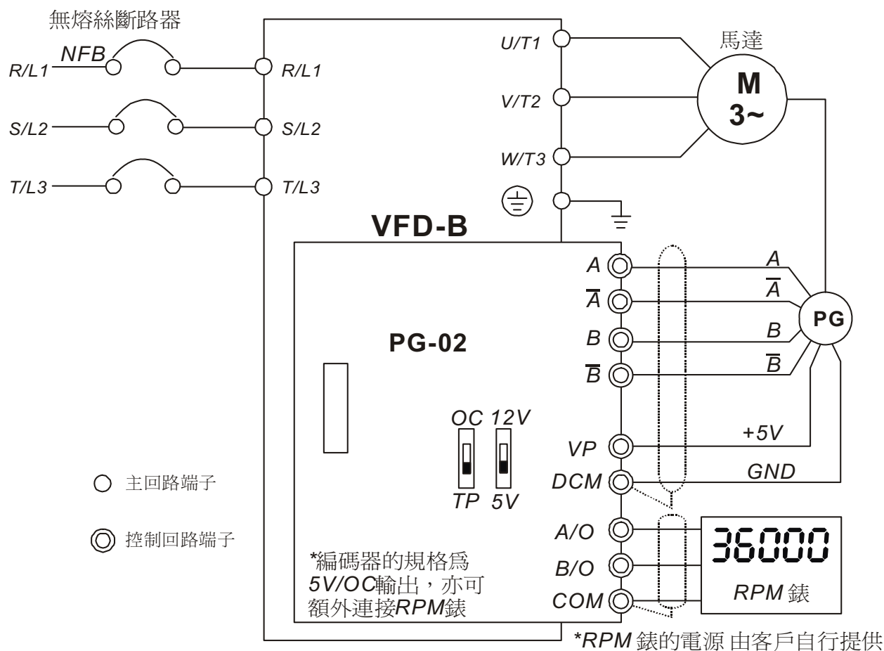
PG-02 與編碼器的連接
