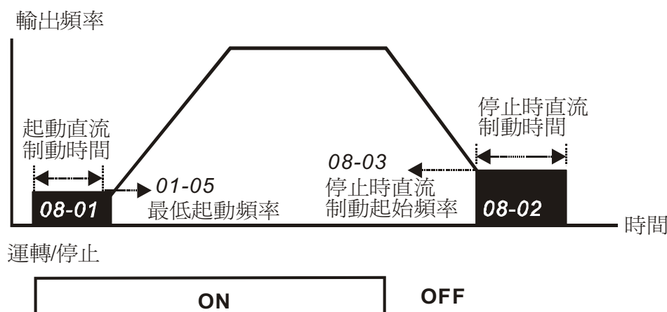
直流制動輸出時序圖
