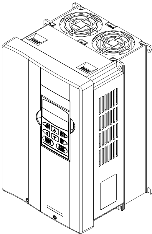
7.5-15HP/5.5-11kW(Frame C)
