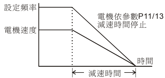
圖一：減速煞車
