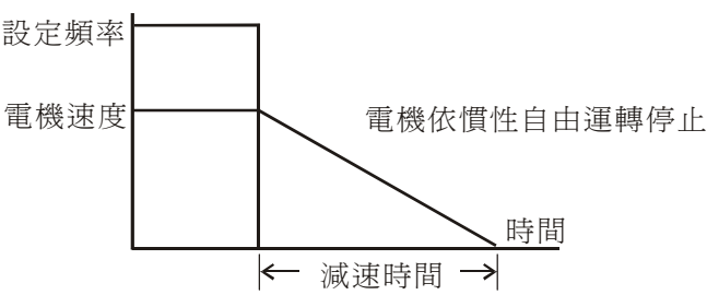
圖二：自由運轉
